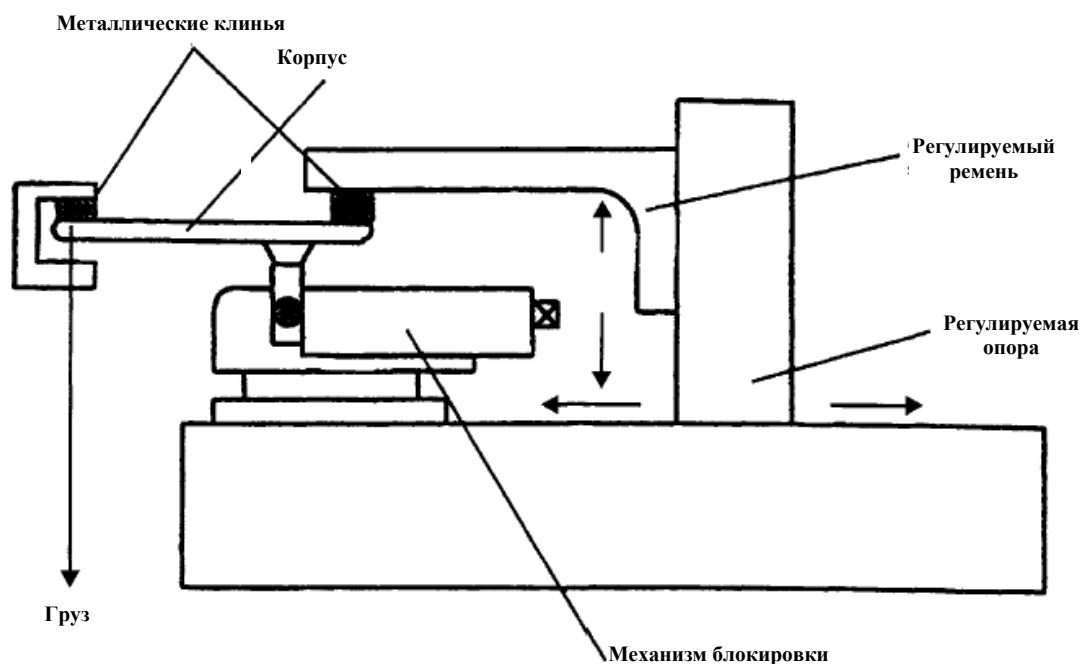
Рис. 3 Пример устройства для испытания на изгиб для зеркал
