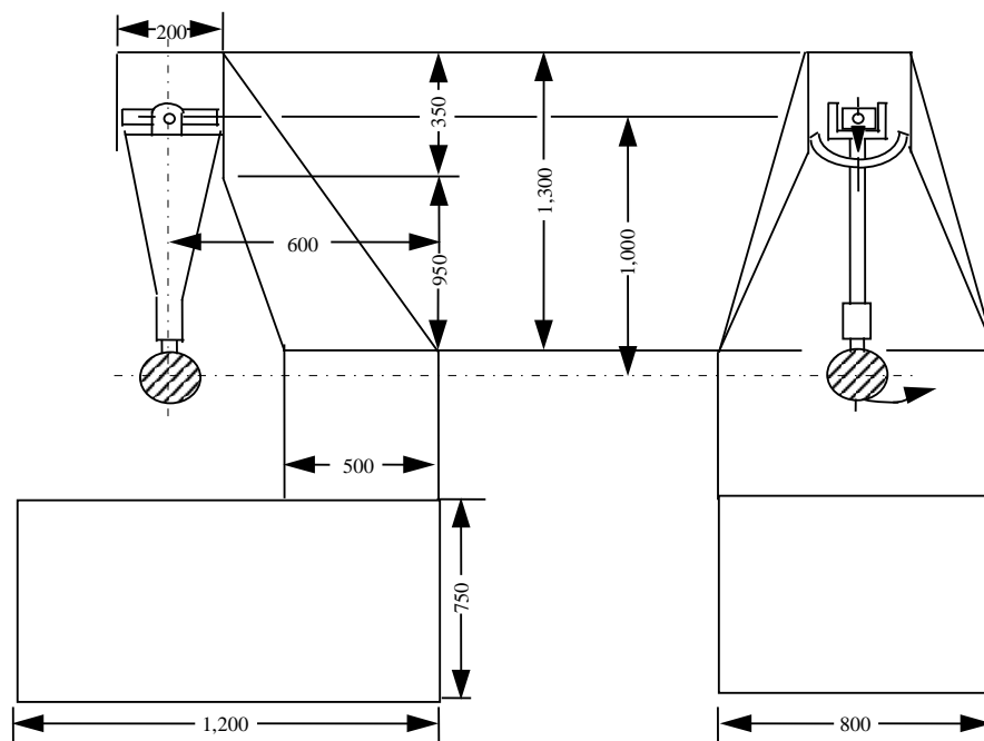
Рис. 2 Размеры испытательного устройства и технические требования (в миллиметрах)
