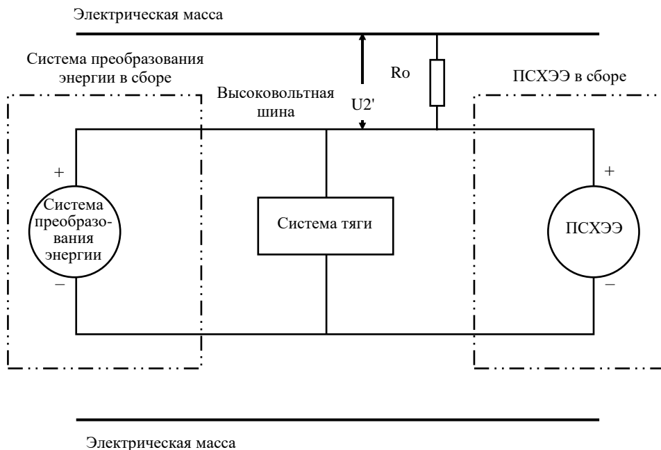
Рис. 6 Измерение U_2'
