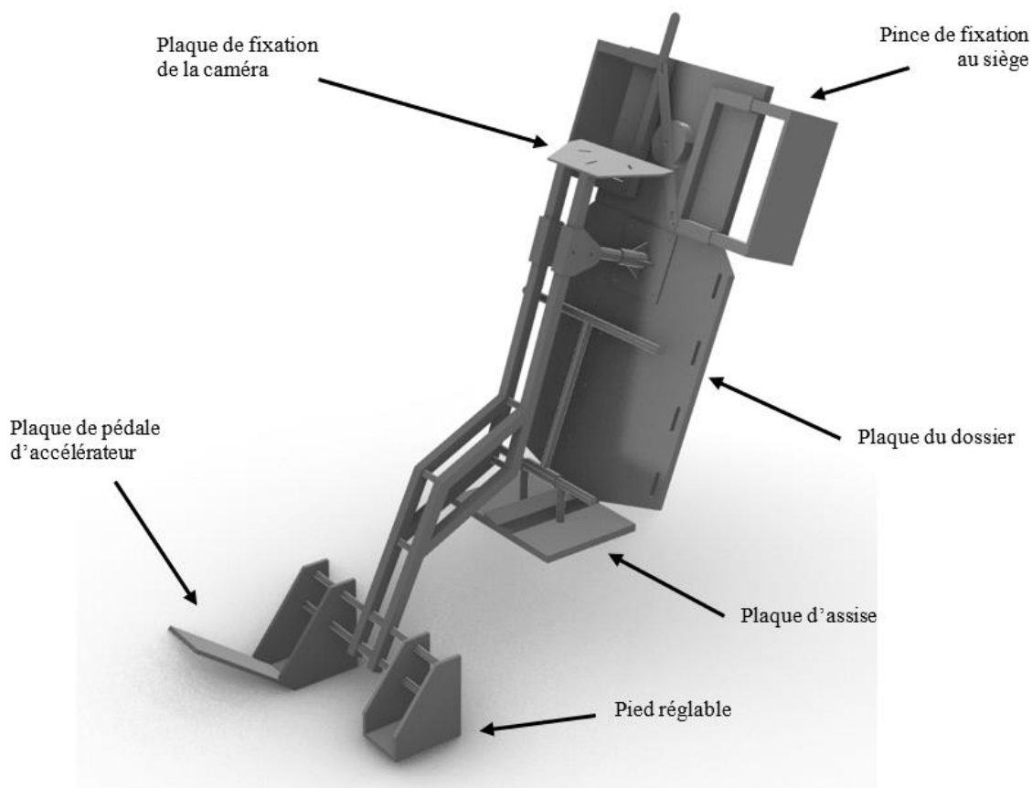
Figure 6 Exemple de dispositif d'essai permettant de positionner des caméras aux points oculaires E1, E2 et E3 préalablement définis
