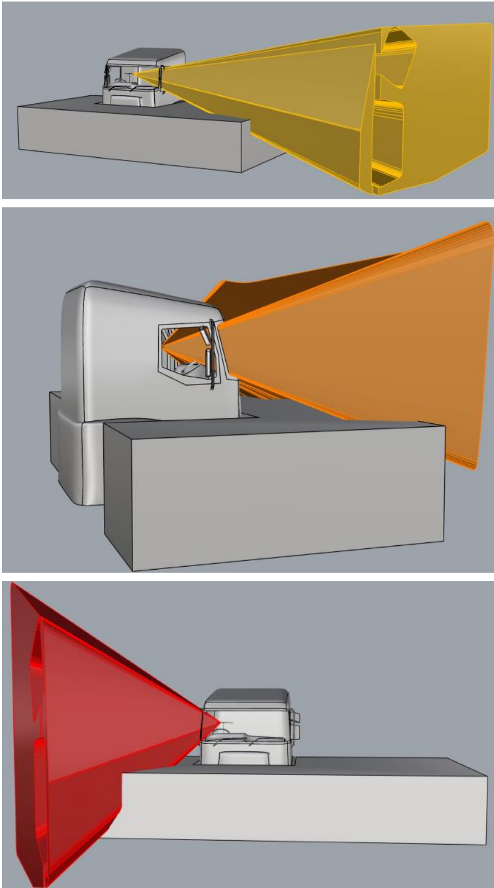
Figure 2 Exemples de vision du conducteur vers la gauche (croquis du haut), vers l'avant (croquis du milieu) et vers la droite (croquis du bas), respectivement projetées à partir des points oculaires E1, E2 et E3 (exemple conçu pour la circulation à gauche)
