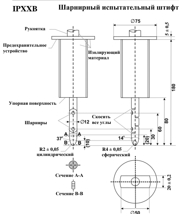
Рис. 3 Шарнирный испытательный штифт
