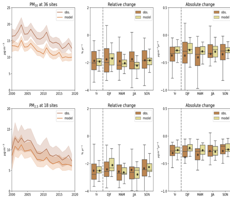
Рис. 5 Наблюдаемые и смоделированные тенденции изменения концентрации PM_{10} и PM_{2.5} за период 2000–2020 годов
