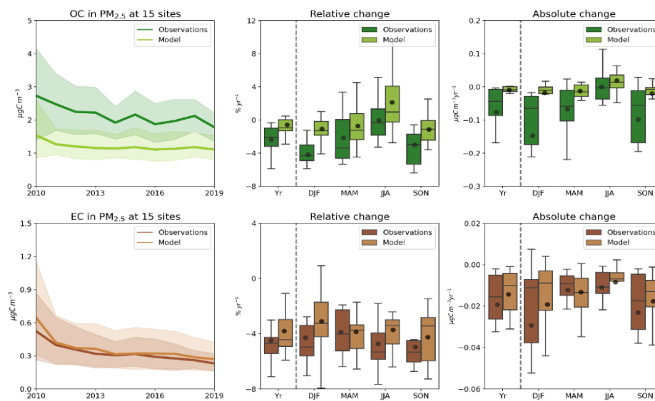
Рис. 6 Наблюдаемые и смоделированные тенденции изменения концентрации органического углерода и элементарного углерода в период 2010–2019 годов
