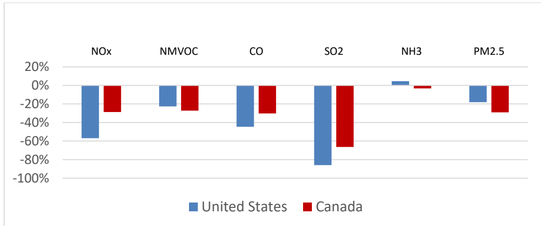
Национальные выбросы Соединенных Штатов Америки (показаны синим цветом) и Канады (показаны красным цветом), изменение за период 2005–2019 годов согласно представленным данным (в процентах)
