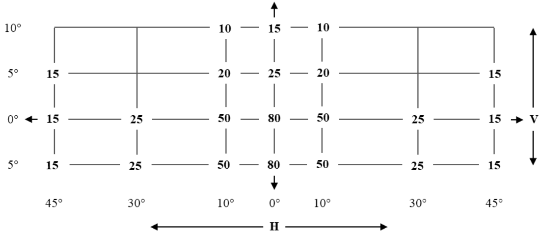
Figure A3-V Répartition de la lumière pour les feux de marche arrière
