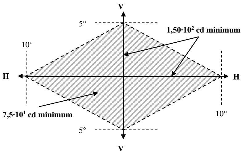
Figure A3-VI Répartition de la lumière pour les feux de brouillard arrière
