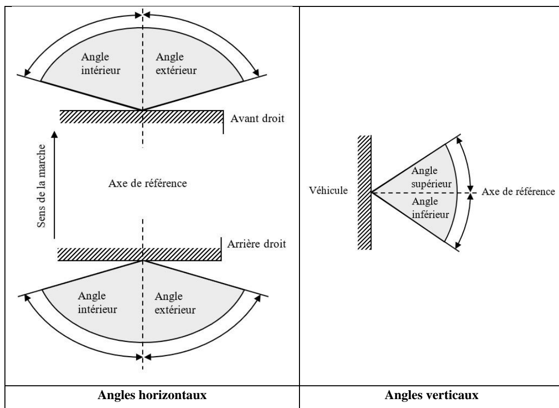
Angles de visibilité géométrique horizontaux et verticaux
