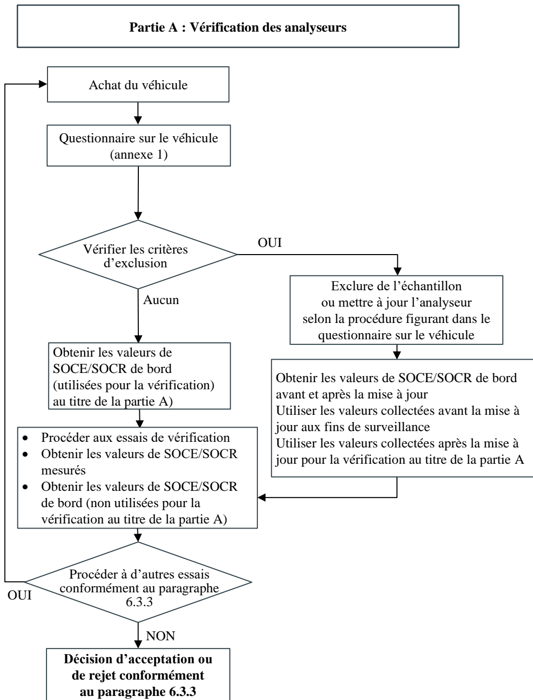
Figure 1 Diagramme de décision pour la partie A : Vérification des analyseurs
