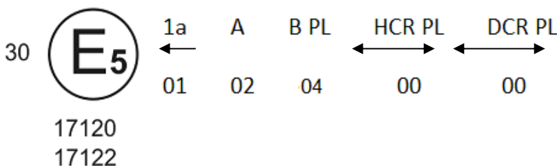
Рис. 4 Огонь, совмещенный с фарой
