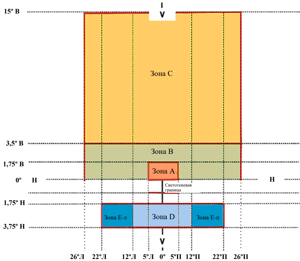
Рис. 2 Распределение света передней противотуманной фары класса В
