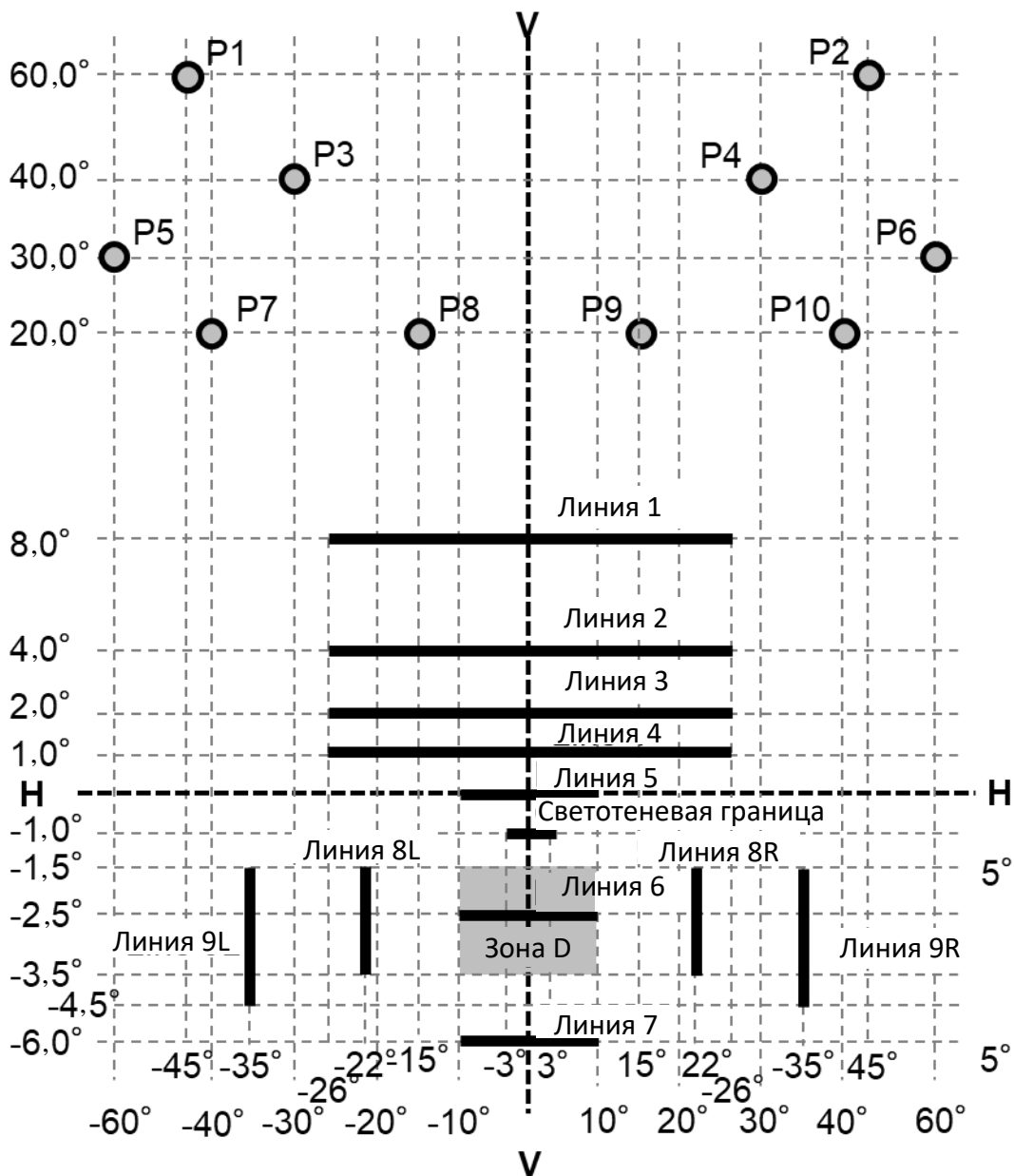
Распределение света передней противотуманной фары класса F3
