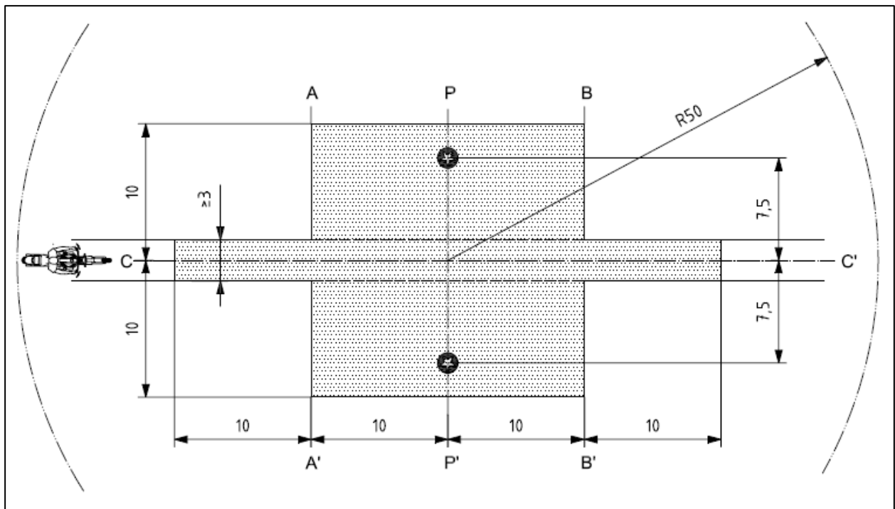
«Рис. 1 Схема испытательного трека с размерами в метрах
