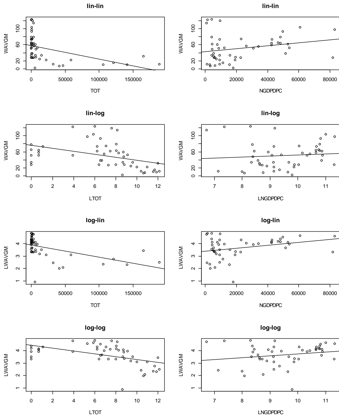
Рис. IX.2 Линии регрессии для данных
