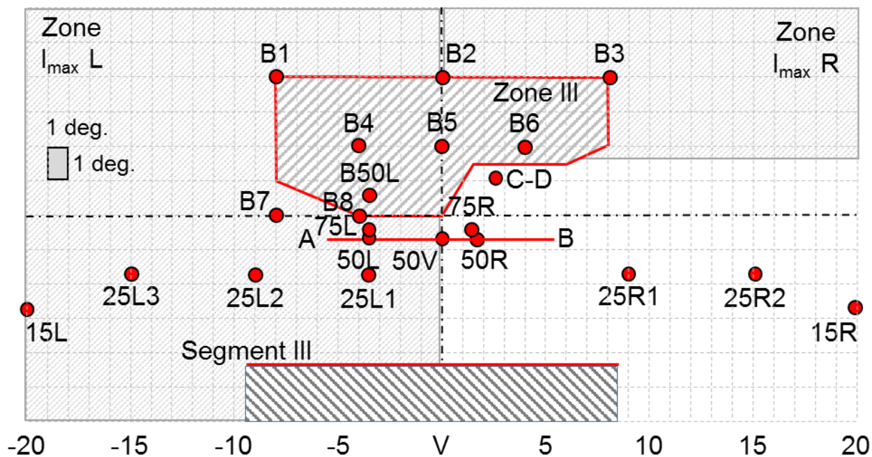
Figure A4-VI Faisceau de croisement équipé de sources lumineuses à décharge conçu pour la circulation à droite
