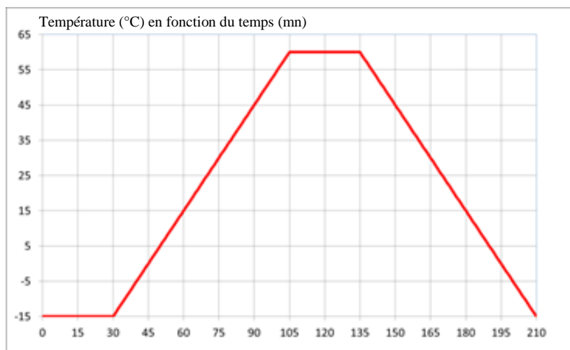
Figure A1/3 Cycle de conditionnement en température
