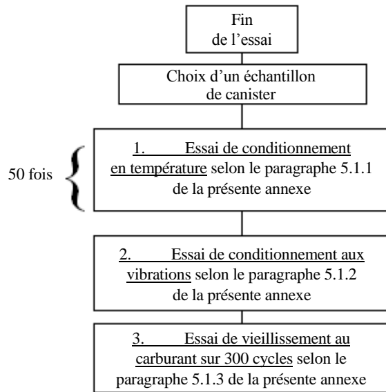
Figure A1/2 Procédure de vieillissement du canister
