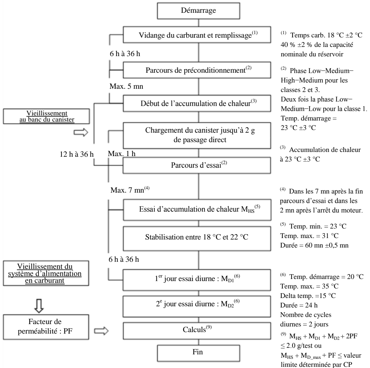
Figure A1/1a Pour les systèmes de réservoirs non totalement étanches
