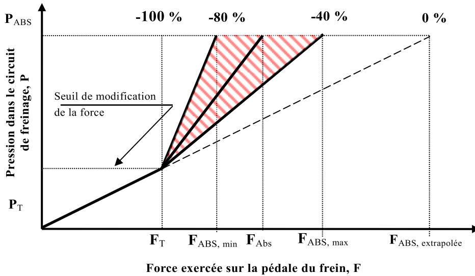
Figure 1b Caractéristique de la force à exercer sur la pédale pour obtenir la décélération maximale avec un système d’assistance au freinage d’urgence de catégorie A
