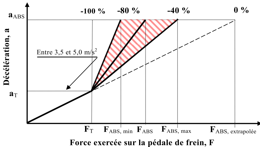
Figure 1a Caractéristique de la force à exercer sur la pédale pour obtenir la décélération maximale avec un système d'assistance au freinage d'urgence de catégorie A
