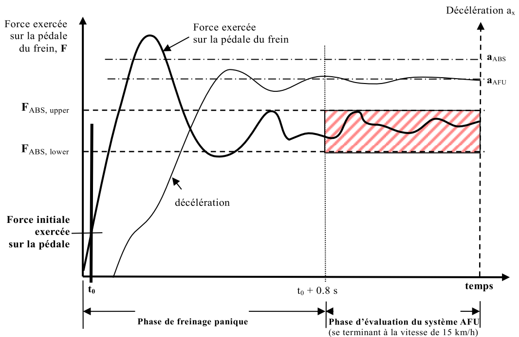
Figure 2 Essai 2 d'un système d'assistance au freinage d'urgence de catégorie B
