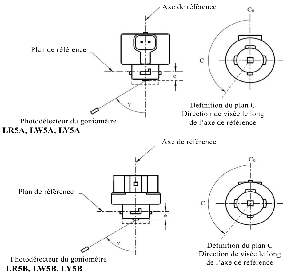
Figure 3 Montage permettant de mesurer la répartition de l'intensité lumineuse
