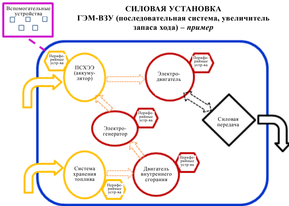
Рис. 5 Гибридный электромобиль – зарядка с помощью внешнего зарядного устройства (последовательная система, увеличитель запаса хода)
