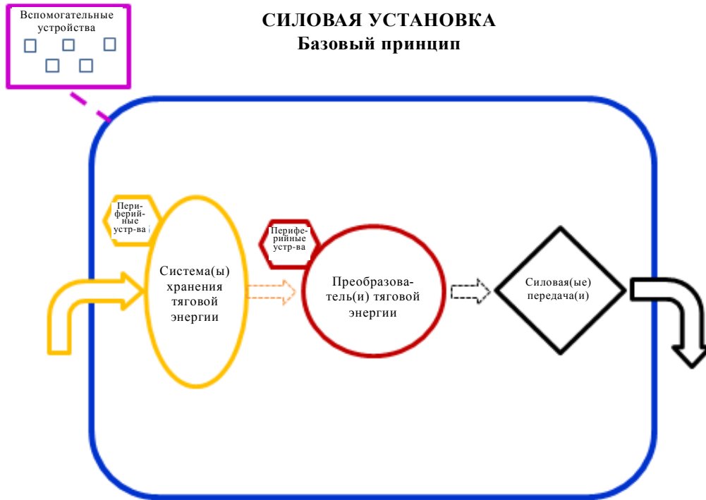
Рис. 1 Силовая установка – базовые принципы
