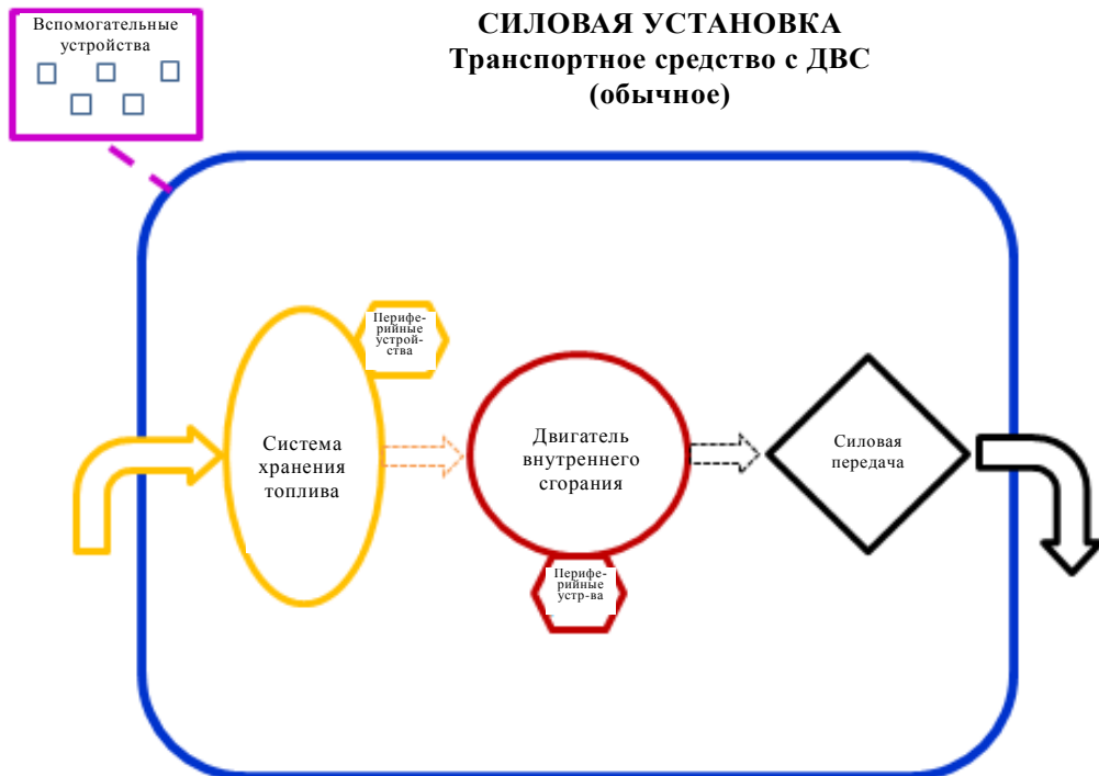
Рис. 2 Транспортное средство с двигателем внутреннего сгорания (обычное)
