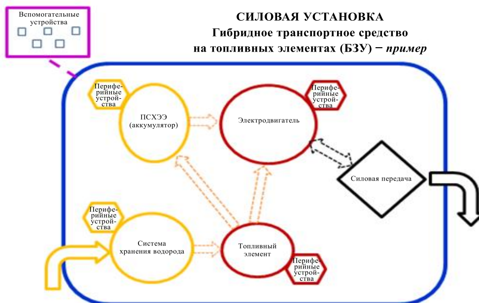
Рис. 7 Гибридное транспортное средство на топливных элементах (зарядка с помощью бортового зарядного устройства)
