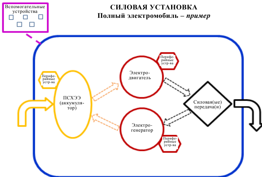
Рис. 3 Полный электромобиль
