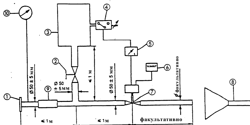
Рис. 3 Испытательное устройство для кондиционирования методом пульсации
