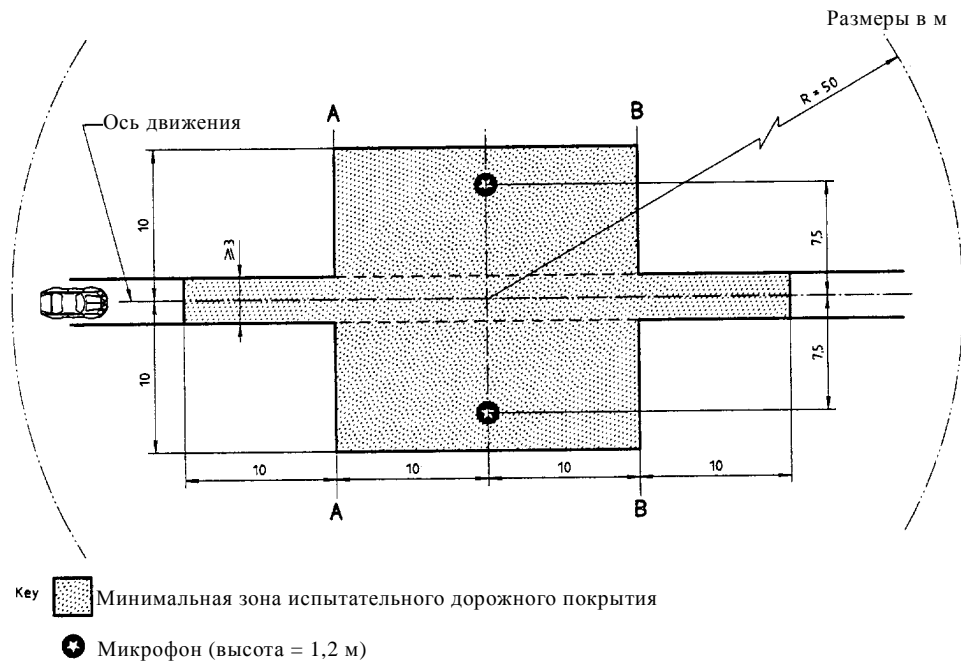
Рис. 1 Минимальные требования к зоне с испытательным дорожным покрытием. Затемненная часть называется "испытательной зоной"
