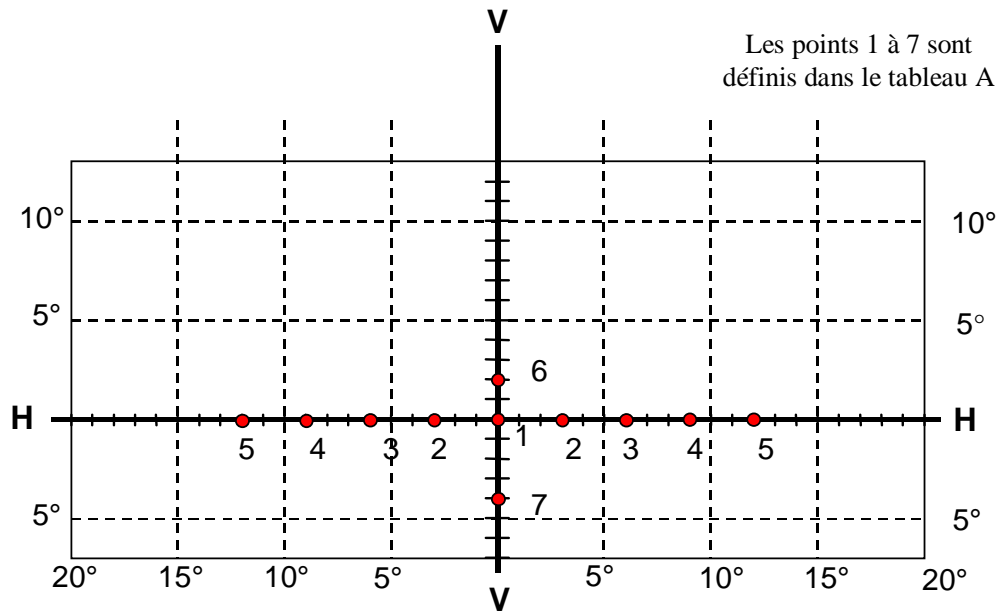
Figure E. Faisceau de route secondaire
