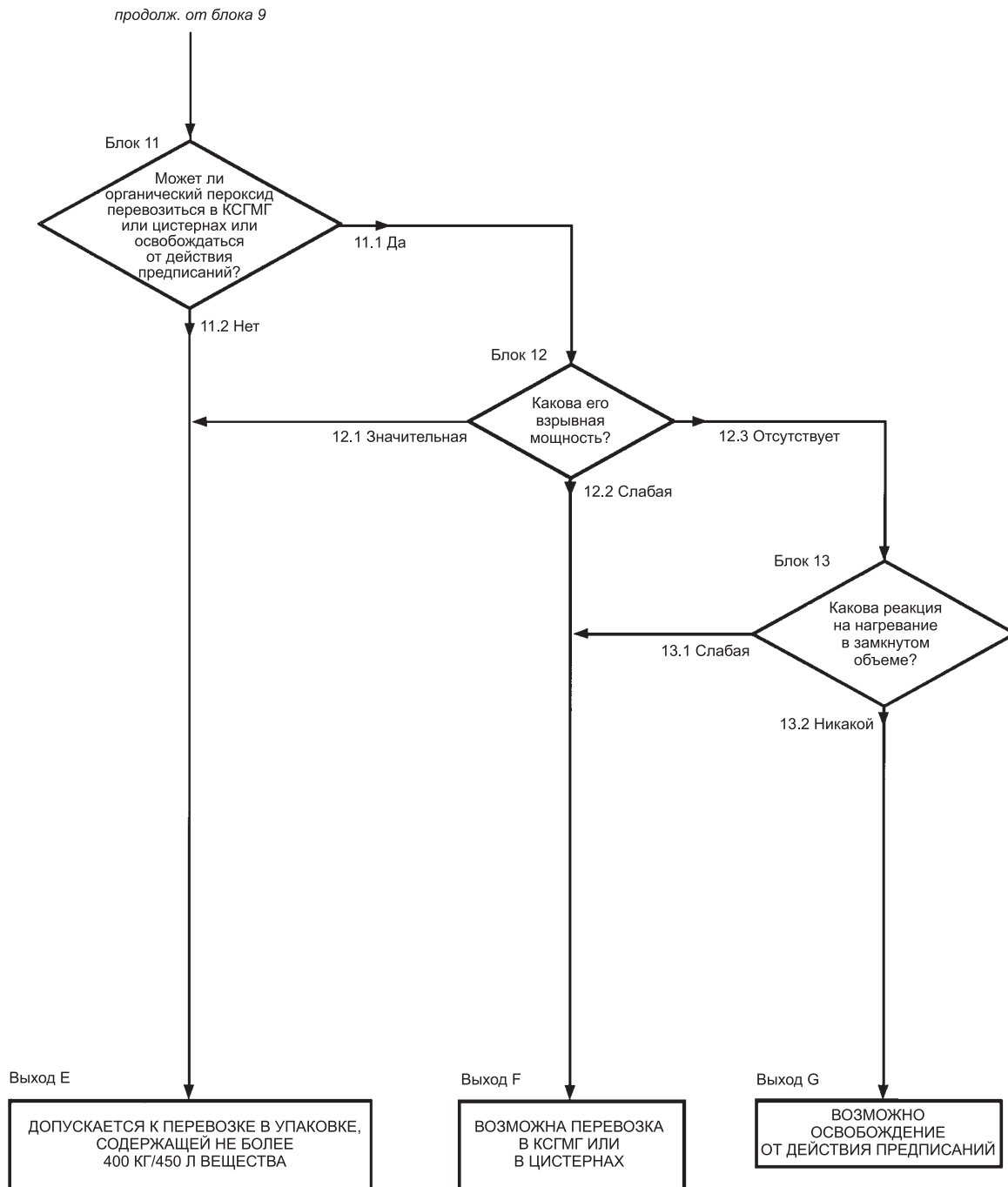
Рис. 2.5.1: СХЕМА ПРИНЯТИЯ РЕШЕНИЯ ОТНОСИТЕЛЬНО УСЛОВИЙ ПЕРЕВОЗКИ ОРГАНИЧЕСКИХ ПЕРОКСИДОВ (продолжение)
