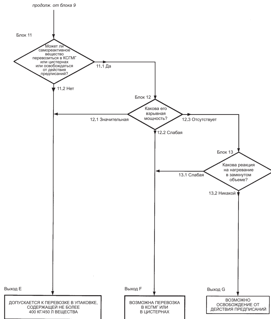
Рис. 2.4.1: СХЕМА ПРИНЯТИЯ РЕШЕНИЯ ОТНОСИТЕЛЬНО УСЛОВИЙ ПЕРЕВОЗКИ САМОРЕАКТИВНЫХ ВЕЩЕСТВ (продолжение)
