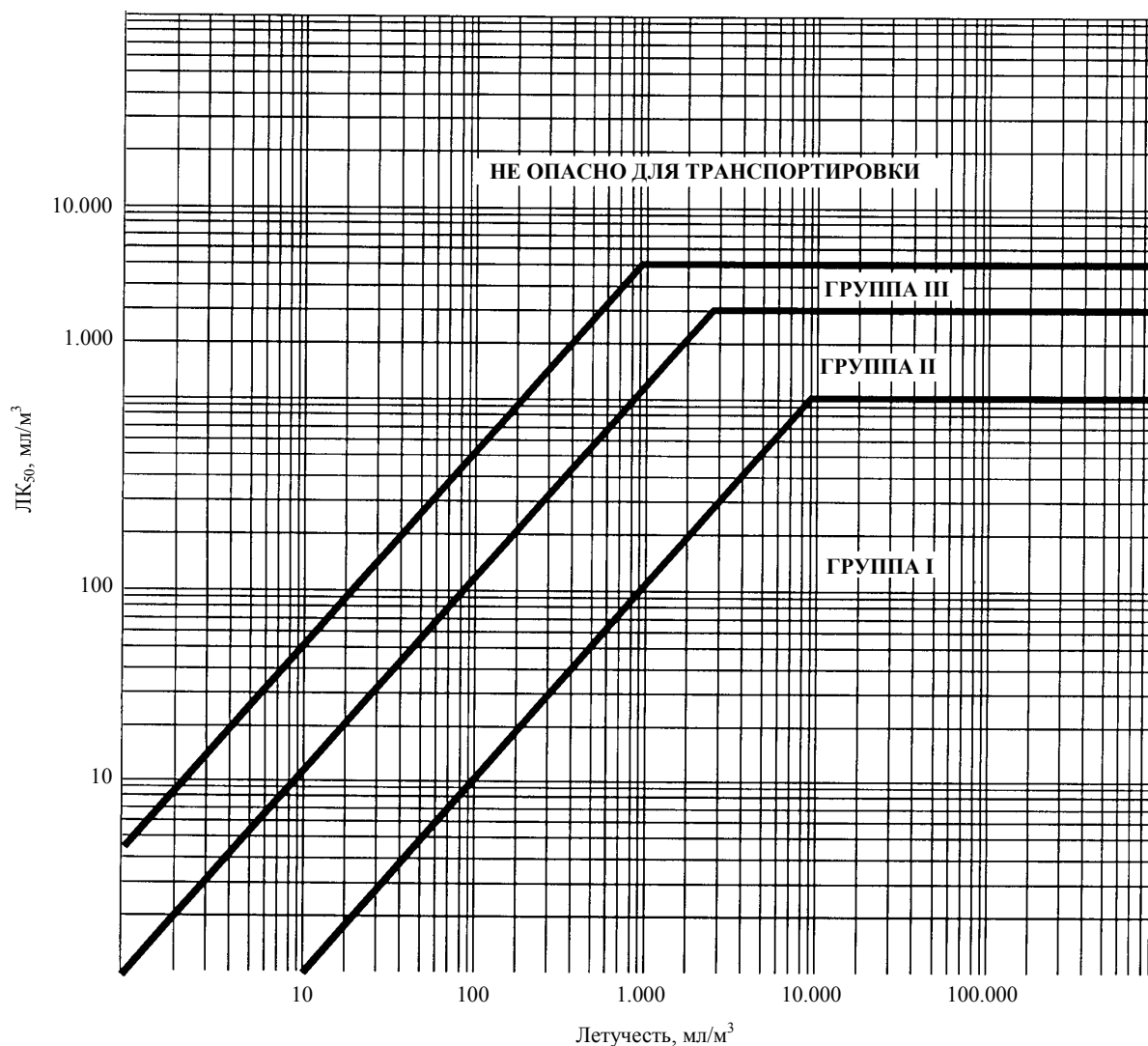
Рис. 2.6.1: ИНГАЛЯЦИОННАЯ ТОКСИЧНОСТЬ: ГРАНИЦЫ ГРУПП УПАКОВКИ
