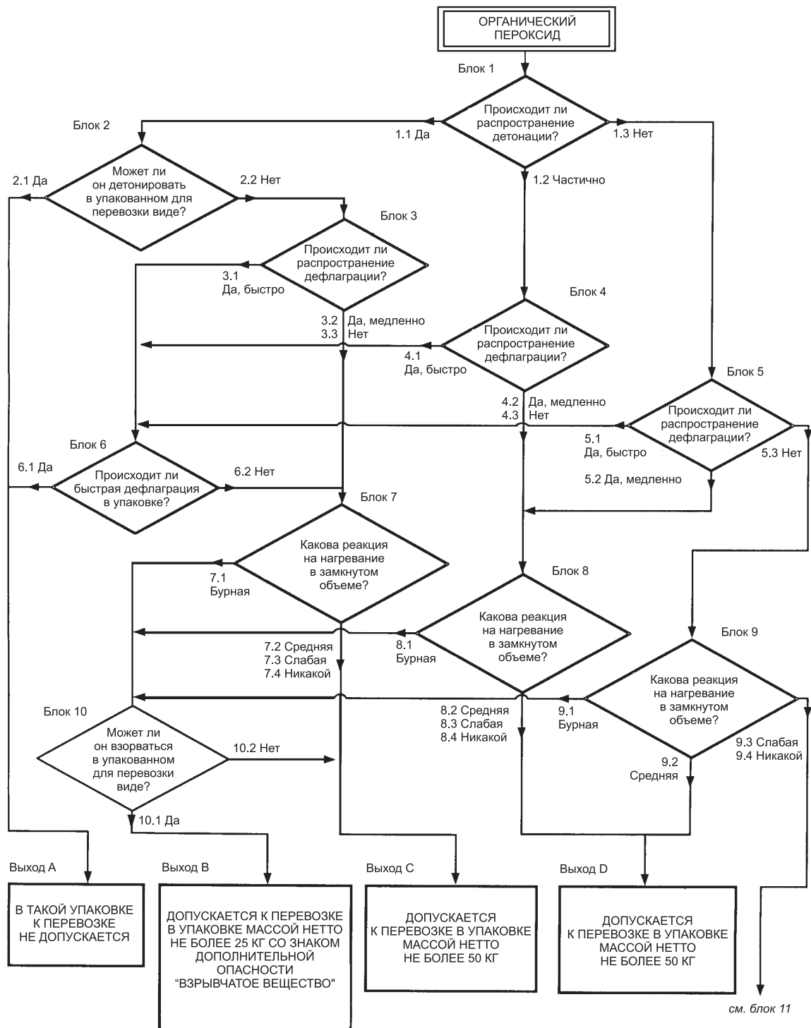
Рис. 2.5.1: СХЕМА ПРИНЯТИЯ РЕШЕНИЯ ОТНОСИТЕЛЬНО УСЛОВИЙ ПЕРЕВОЗКИ ОРГАНИЧЕСКИХ ПЕРОКСИДОВ
