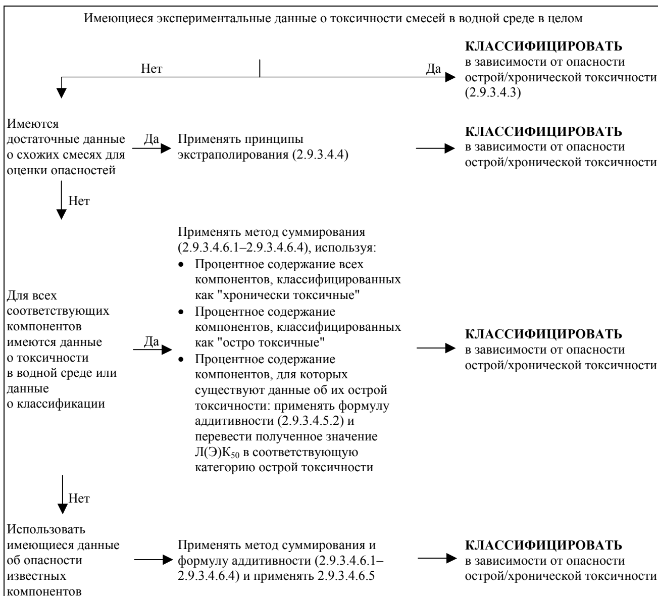
Рис. 2.9.1: Ярусный подход к классификации смесей в зависимости от их острой и хронической токсичности в водной среде
