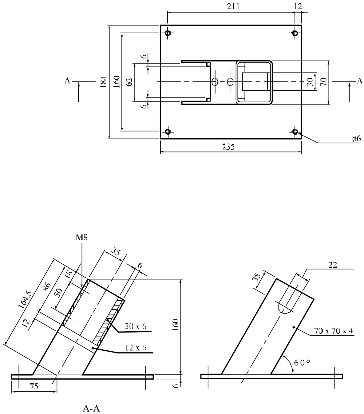
Рис. 11.6.1.2: ОПОРНЫЙ СТЕНД
