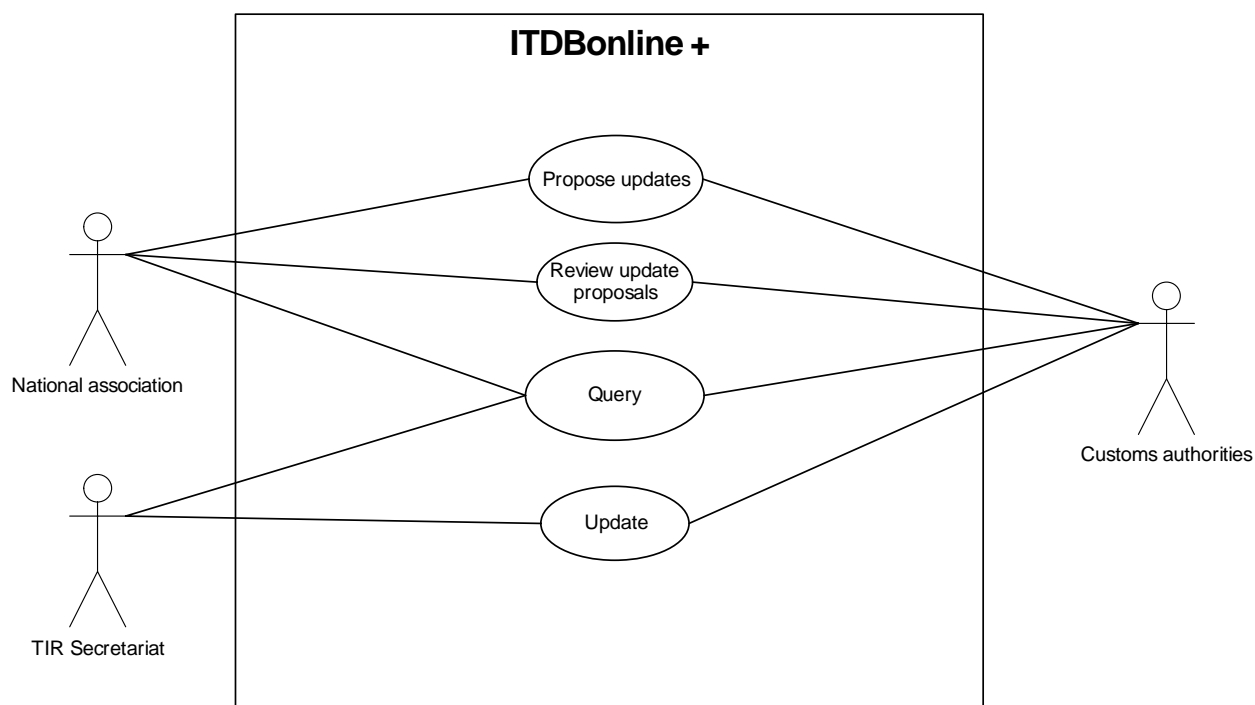
Рис. 4 – Схема варианта использования высокого уровня (только на английском языке)
