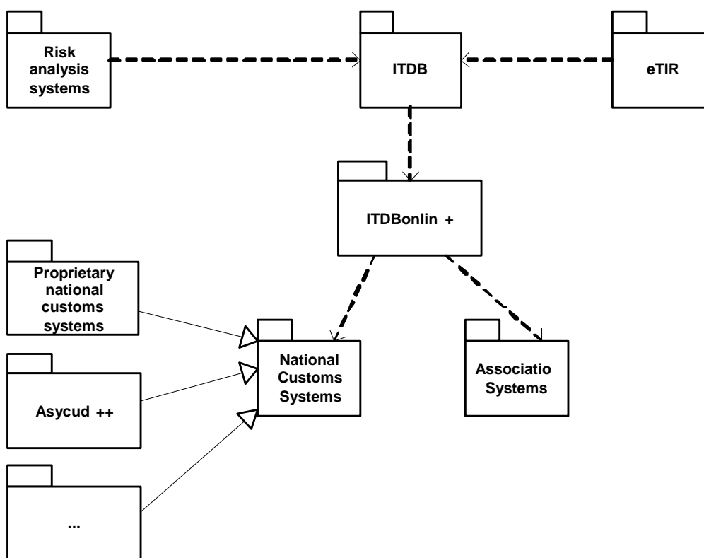
Рис. 3 – Схема общего пакета (только на английском языке)
