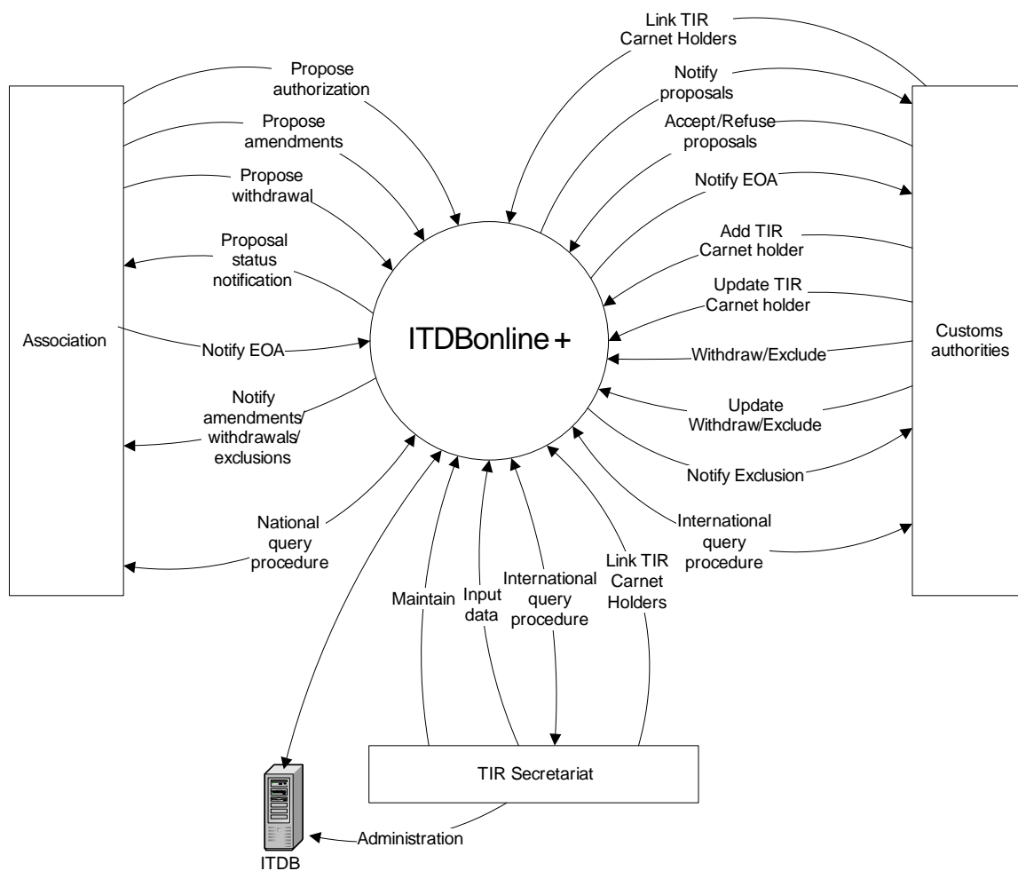
Рис. 2 - Схема бизнес-контекста "МБДМДПонлайн+" (только на английском языке)
