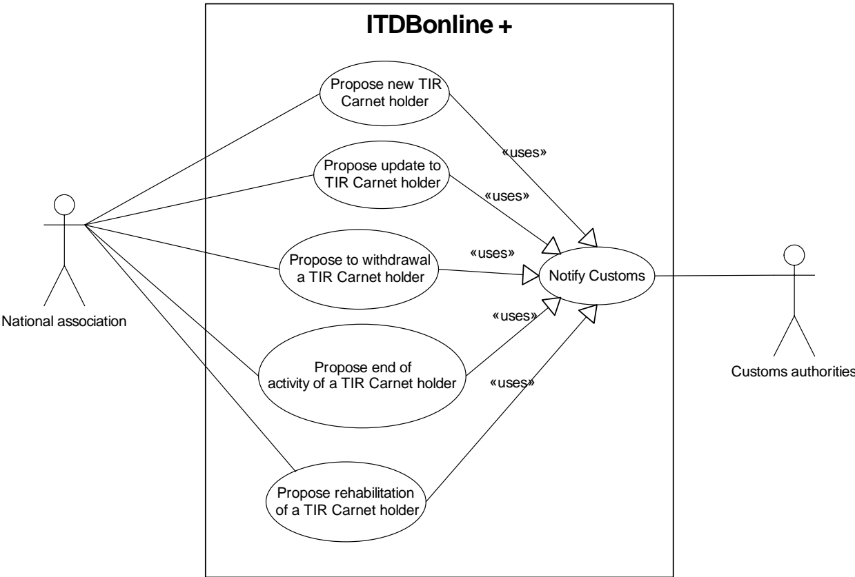
Рис. 5 – Схема варианта использования для внесения предложений об обновлениях (только на английском языке)
